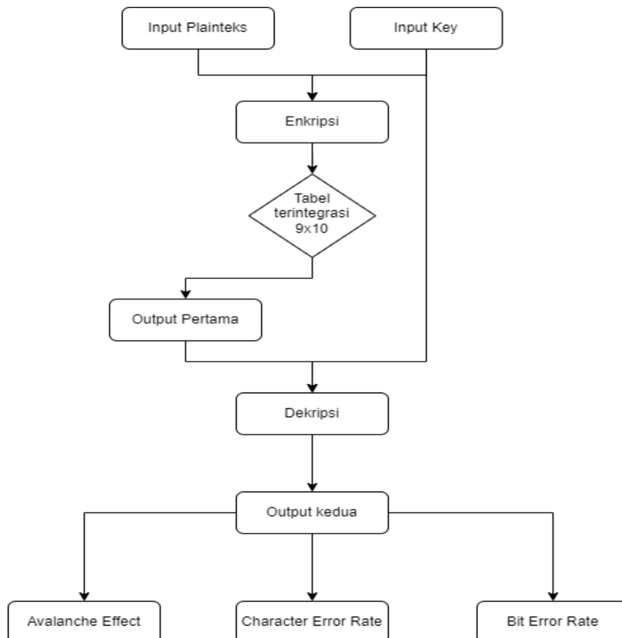
Gambar 2. Flowchart Playfair Cipher ASCII dengan Tabel Matriks 9x10
